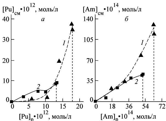
Рис. 3. Изотермы сорбции Pu (а) и Am (б) на смоле КБ-4: 1 – для системы с дерновой супесчаной почвой, 2 – для системы с дерново-подзолистой песчаной почвой. [Pu, Am] см – концентрация радионуклидов на смоле, [Pu, Am] р – в растворе.
