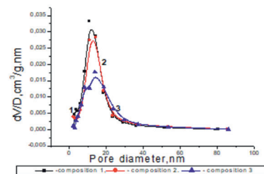
Адсорбционные свойства
