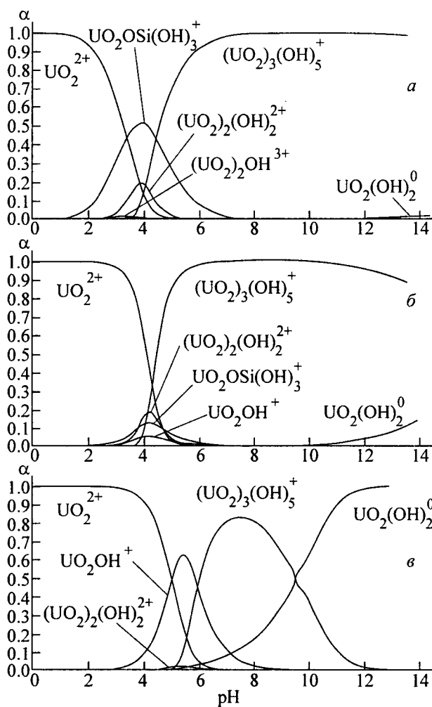
Рис. 2. Формы нахождения U(VI) в водном растворе.
