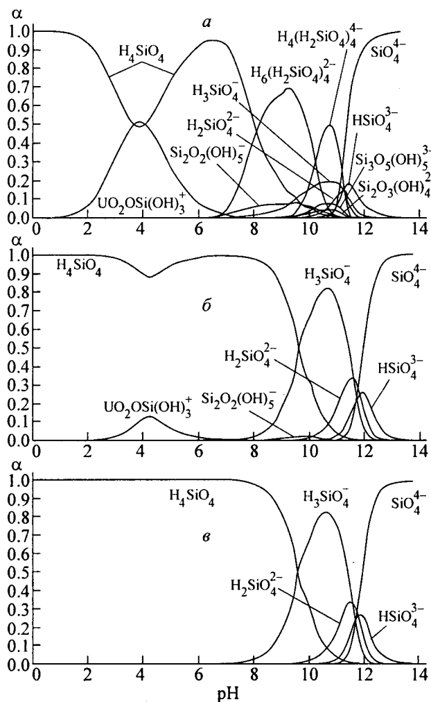
Рис. 1. Формы нахождения Si(IV) в водном растворе. а - C_{Si} = C_U = 1 \cdot 10^{-1} моль/л; б - C_{Si} = C_U = 1 \cdot 10^{-3} моль/л; в - C_{Si} = C_U = 1 \cdot 10^{-6} моль/л; \alpha - мольная доля соответствующей ионно-молекулярной формы в растворе; то же для рис. 2.
